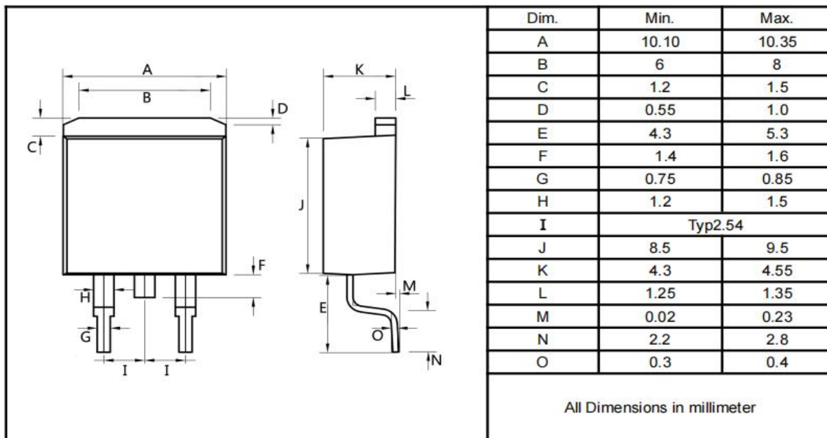
TO-263
